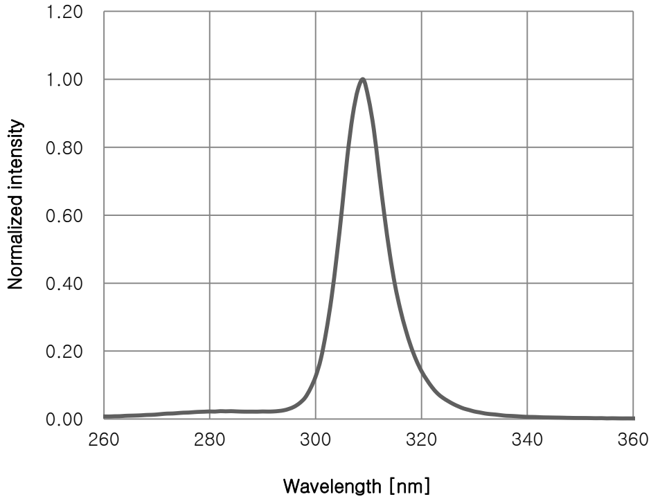
Fig 1. Spectrum, T_a=25^\circ\text{C} , I_F=600\text{mA}
